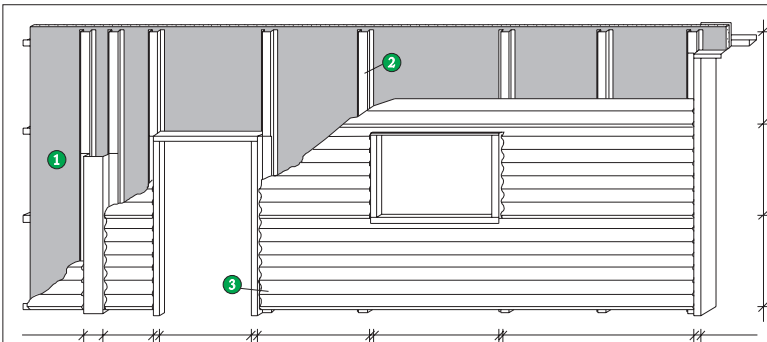
Fasado brėžinys
